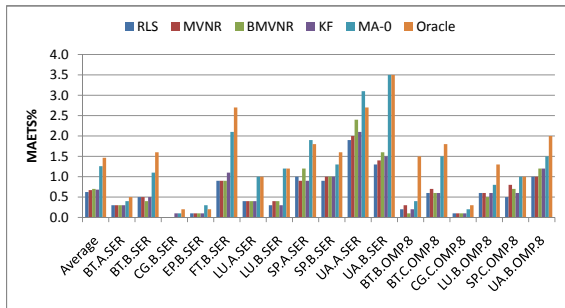
(b) MAETS
